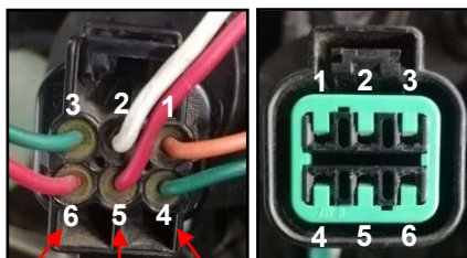
Задний разъем (6 PIN)
