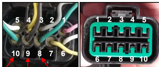
Złącze przednie (10 PIN)
