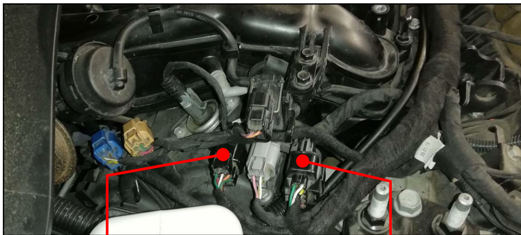
Złącze tylne (6 PIN)
