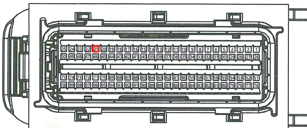
Złącze B (ECU)
