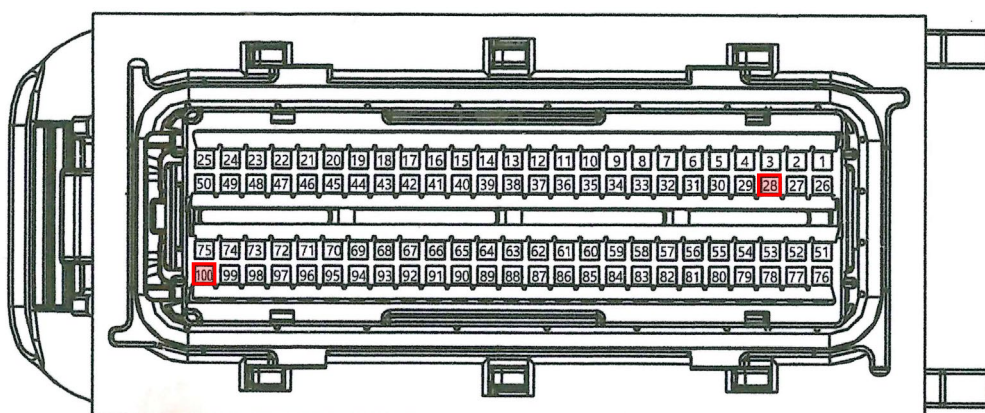
Złącze A (ECU)
