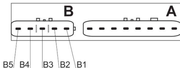
WIDOK ZŁĄCZ WIĄZKI STEROWNIKA WTRYSKIWACZY BENZYNOWYCH
