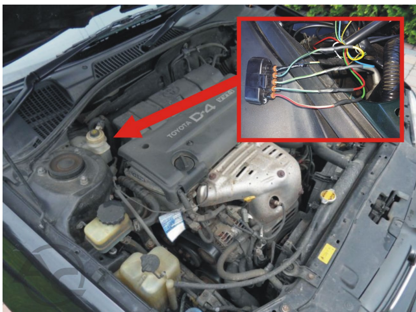
Вид разъемов жгута контроллера бензиновых инжекторов.
