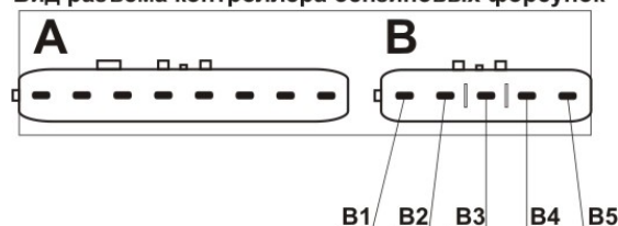
РАЗЪЁМ А РАЗЪЁМ В Вид разъёма контроллера бензиновых форсунок
